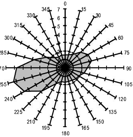
Øyra (bunndyp - 67m) Gjennomsnittshastighet (cm/s)
