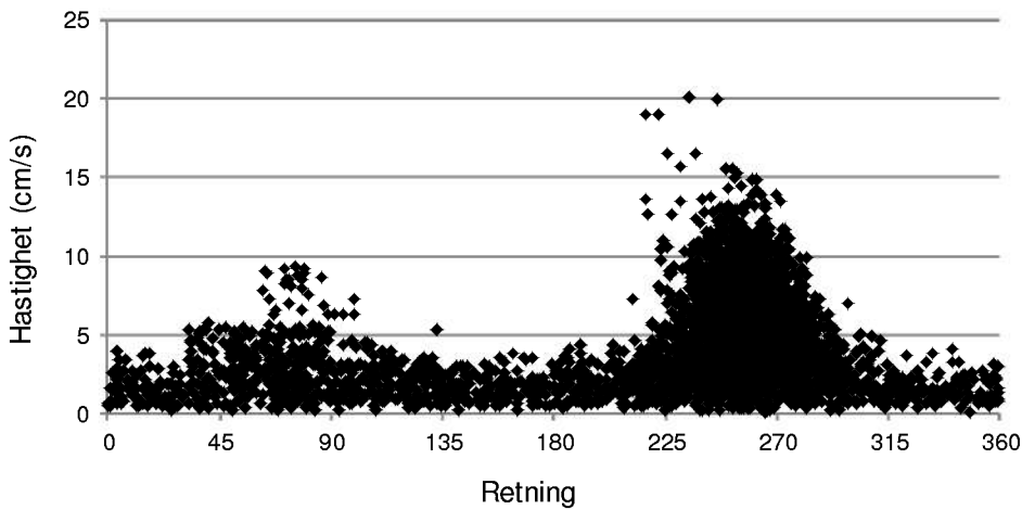
Øyra (bunndyp - 67m)
