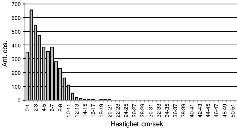
Øyra (bunndyp - 67m)
