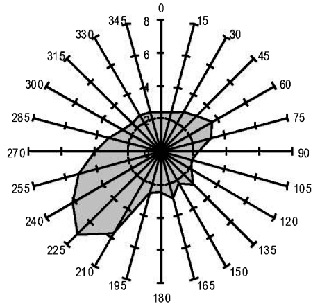
Øyra (spredningsdyp - 42m) Gjennomsnittshastighet (cm/s)
