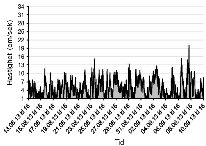
Øyra (bunndyp - 67m)
