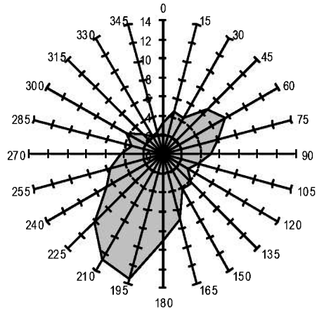
Øyra (15m dyp) Gjennomsnittshastighet (cm/s)
